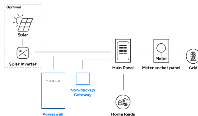
Рис. 1 – Структурна схем підключення Tesla Powerwall
