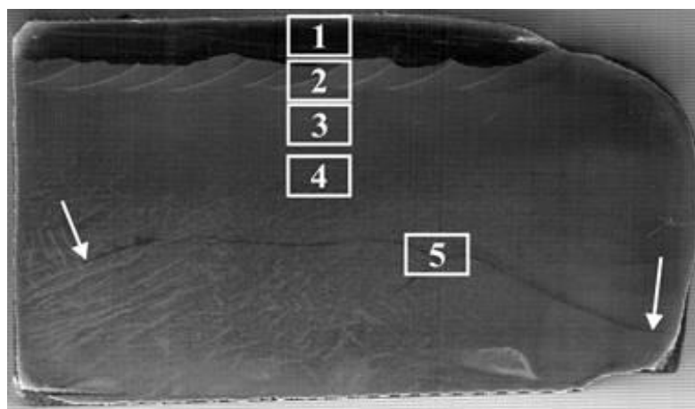
Рис. 1 – Макроструктура зразка (×1)
