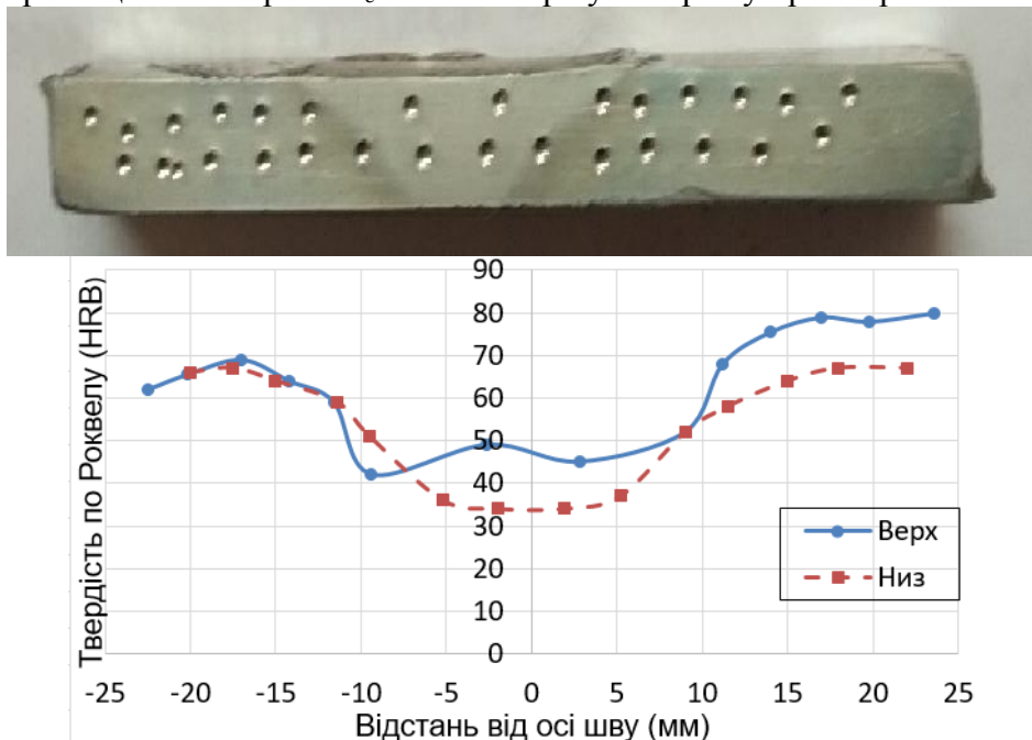
Рис. 1 – Розподіл твердості по Роквелу в з'єднанні ЗТП пластин зі сплавом A2219-T81
