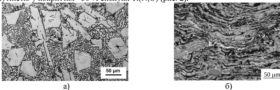
Рис. 2 – Мікроструктура литого евтектичного сплаву та детонаційного покриття
