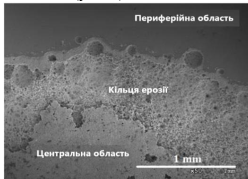
Рис. 3 – Вплив крайового ефекту на зразки сталі AISI 440B азотовані в плазмі аномального тліючого розряду (збільшення \times 50 ) [2]
