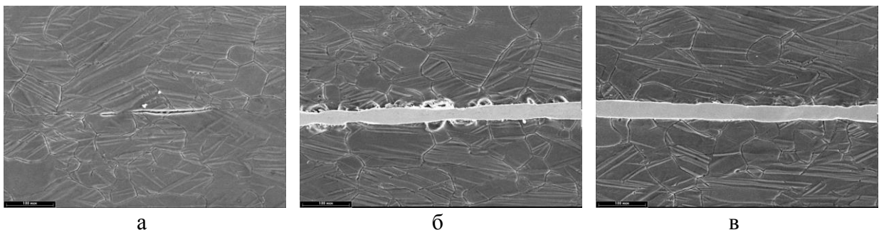
Рис. 1 – Мікроструктура зварних з'єднань зі сплаву МА2, отриманих у формуючих матрицях без (а) і через проміжний прошарок з Ni (б) та Ti (в) на режимі: T_{зв} = 420\text{ }^{\circ}\text{C} , P_{зв} = 10\text{ МПа} , t_{зв} = 30\text{ хв}
