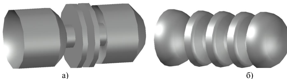
Рис. 1 – Геометрична модель циліндрично-двотискового а) та манжетно-чашкового б) очисного поршня
