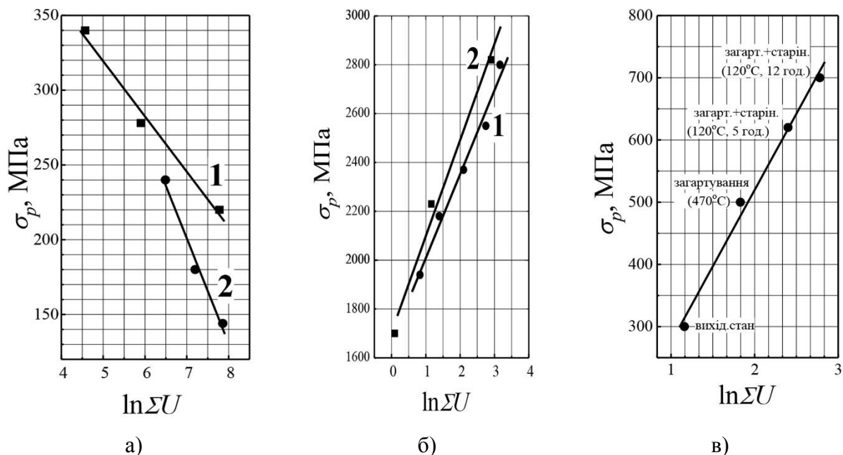
Рис. 1 – Залежність межі міцності зразка \sigma_p від величини середньої сумарної амплітуди \sum U при індентуванні:
