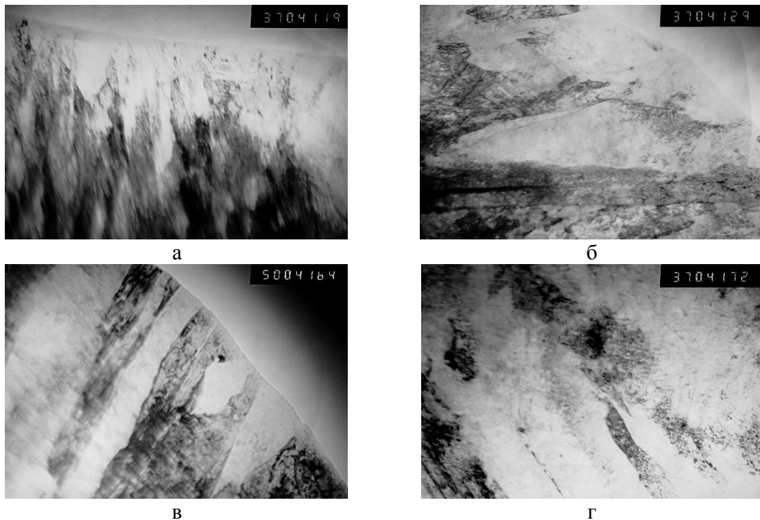
Рис.1 – Тонка (М-А) структура по глибині від обробленої поверхні сталі 4Х5МФ1С після імпульсно-плазмової обробки: а – оброблена поверхня режим I ( \times 37000 ); б – перехідна зона ( \delta від 40 до 70 мкм) режим I ( \times 37000 ); в – оброблена поверхня режим II ( \times 50000 ); г – перехідна зона ( \delta від 25 до 70 мкм) режим II ( \times 37000 ).
