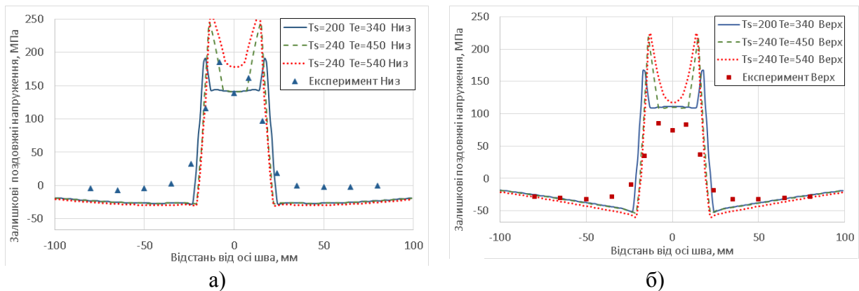
Рис. 4 – Результати моделювання розподілу залишкових поздовжніх напружень на нижній (а) і верхній б) поверхнях з'єднання ЗТП
