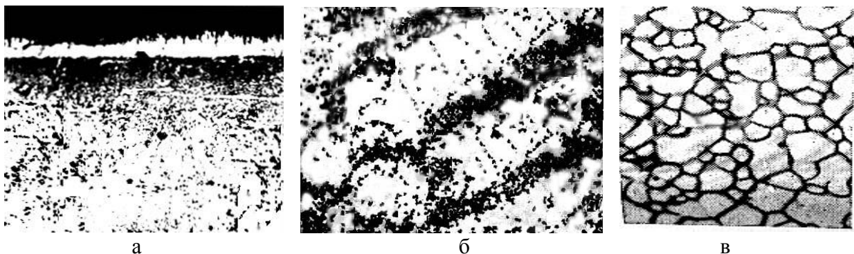
Рис. 2 – Розподіл ^{63}\text{Ni} в залізі після осадження на пресі зі швидкістю = 4 \cdot 10^{-4} \text{ с}^{-1} (вздовж напрямку дифузії, \times 300 ) (а), розтягування = 3 \cdot 10^{-3} \text{ с}^{-1} (у площині, паралельній поверхні, на глибині \sim 10 \text{ мкм} , \times 2500 ) (б), дифузійного зварювання 1 \cdot 10^{-2} \text{ с}^{-1} (на відстані \sim 15 \text{ мкм} від зварного шва, \times 200 ) (в)
