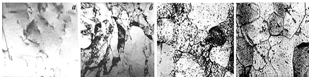
Рис. 4 – Структура Fe у вихідному стані ( a – \times 20000 , б – \times 300 ) і після УЗ ( б – \times 20000 , г – \times 300 ).
